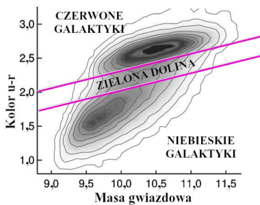
Rys. 1. Diagram kolor-masa gwiazdowa przedstawiający różne typy galaktyk. Kolor tworzy różnicę energii zaobserwowanej w pasmach obserwacyjnych u oraz r . Galaktyki gwiazdotwórcze są niebieskie i znajdują się głównie w lewym dolnym rogu diagramu, natomiast galaktyki martwe i czerwone znajdują się w górnej połowie diagramu. Zielona dolina, zaznaczona liniami, jest obszarem przejściowym, w którym znajduje się stosunkowo niewiele galaktyk. Wykres zaadaptowany z pracy Schawinski et al., 2014.
