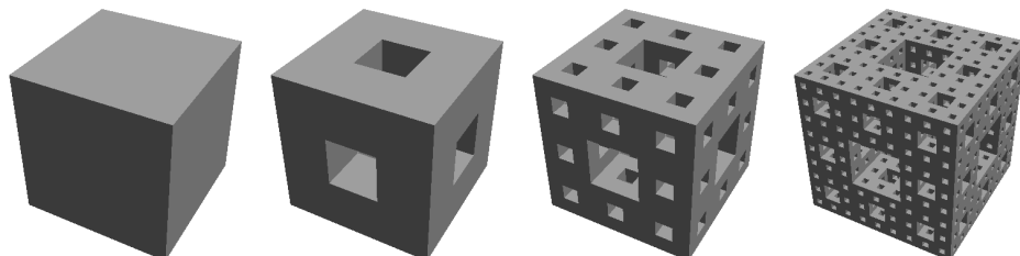
Rys. 2. Trzy początkowe kroki konstrukcji kostki Menger (Wikimedia Commons, autor: Mattcomm)
